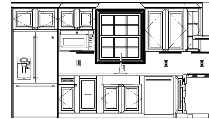
Elevation 2
